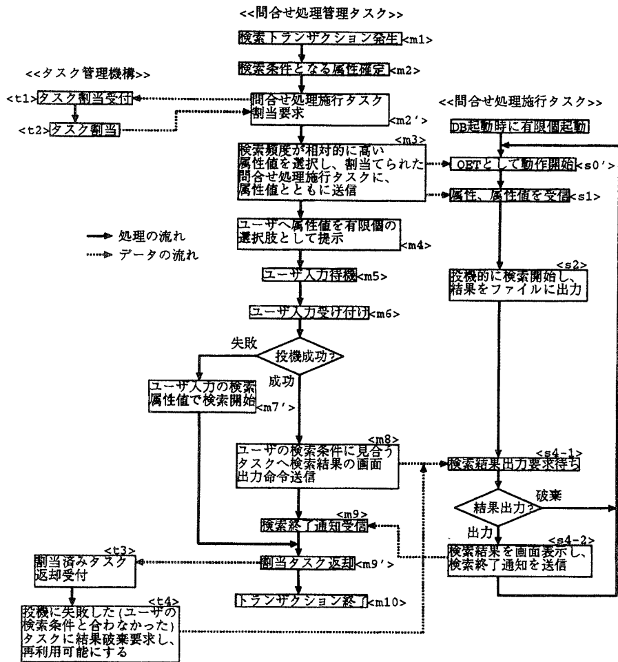
図 3: 静的起動方式のアルゴリズム
