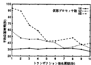
(a) 応答時間だけに注目したもの
