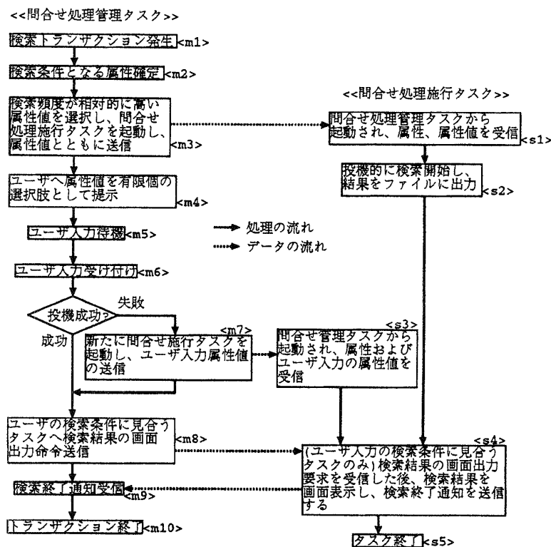
図 2: 動的起動方式のアルゴリズム
